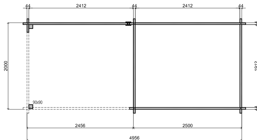
Plattegrond / Plan
